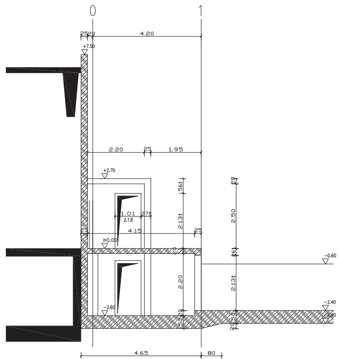
Schnitt A-A
