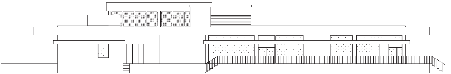
ANSICHT WEST
