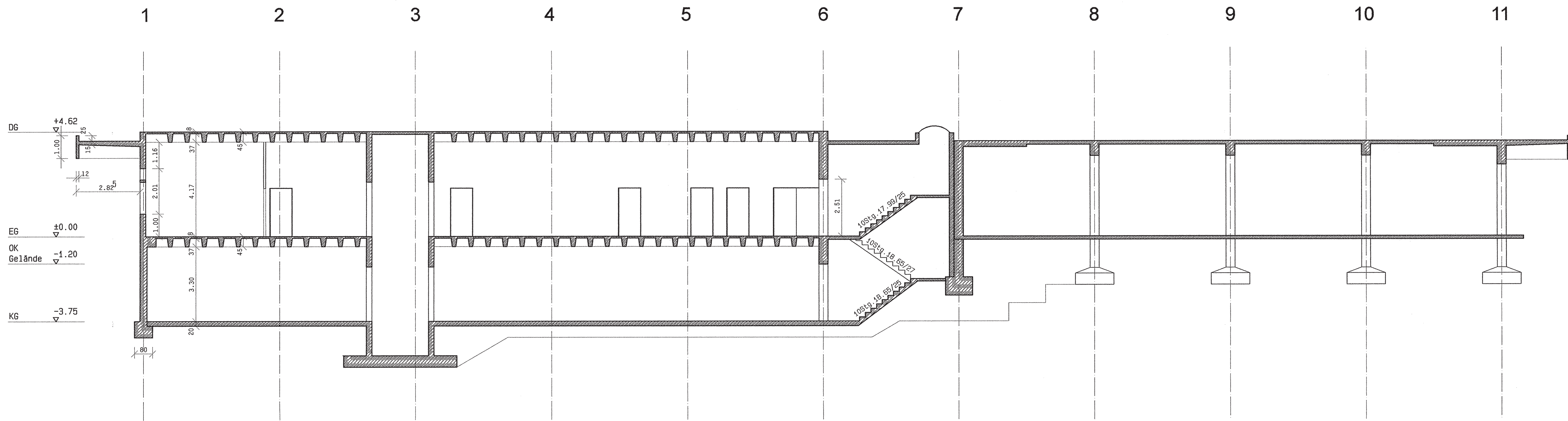
Schnitt A-A
