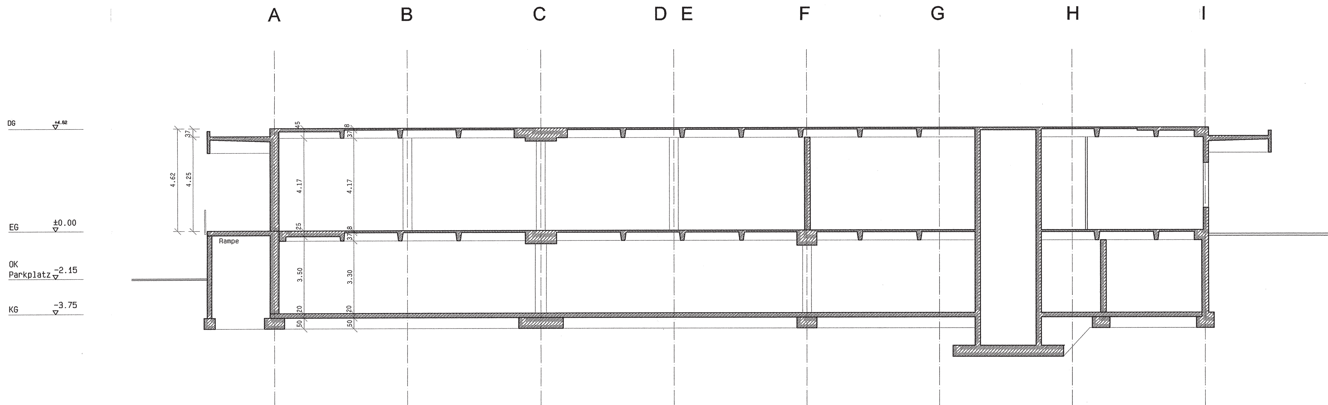
Schnitt B-B
